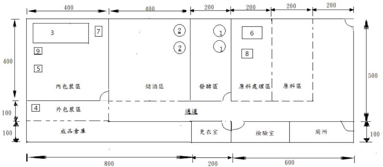
三三製酒行廠房設備比例配置圖 比例尺：1:100 單位：mm
